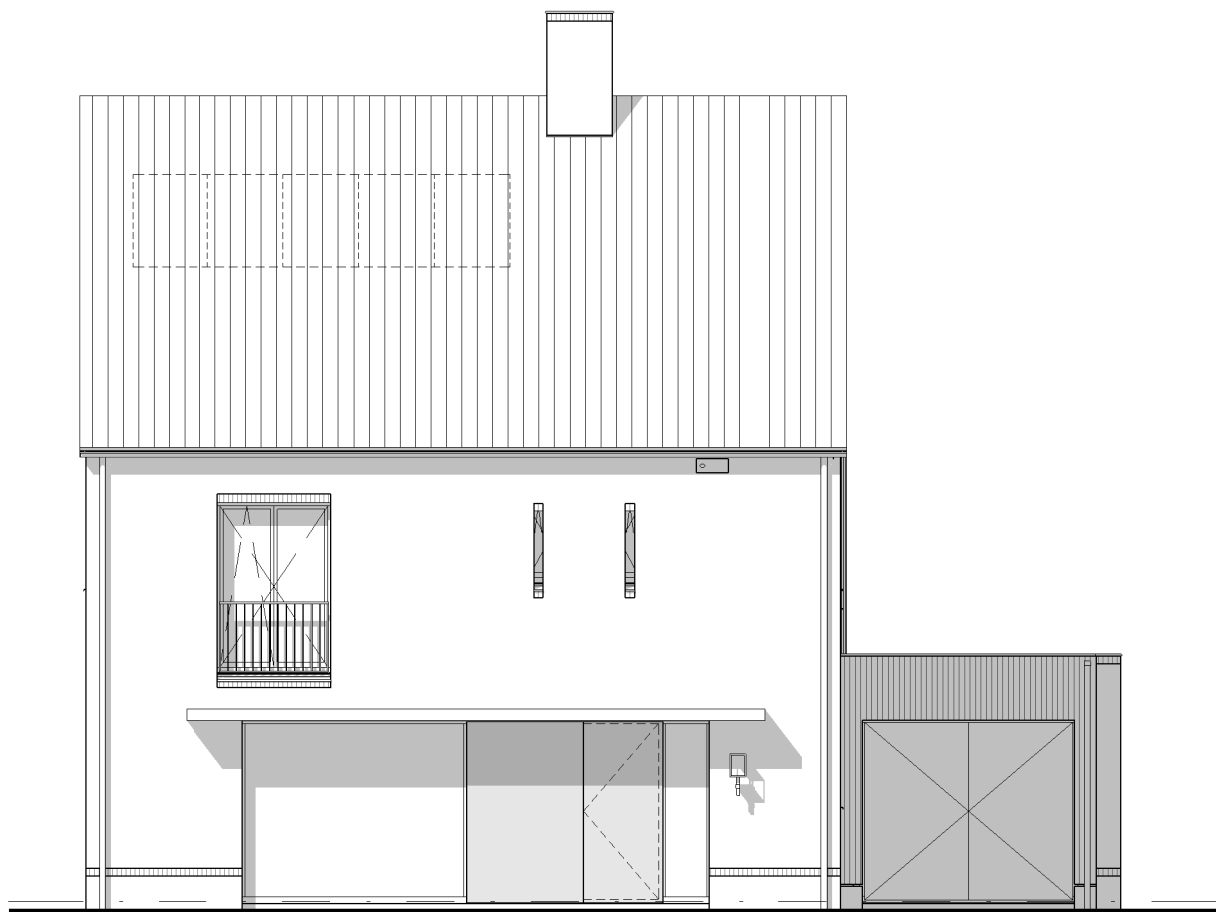
VOORGEVEL
